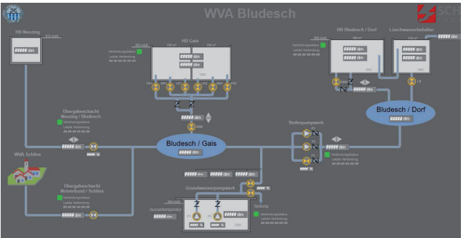
Konzept-Übersicht Prozessleitsystem für die Wasserversorgung in Bludesch
